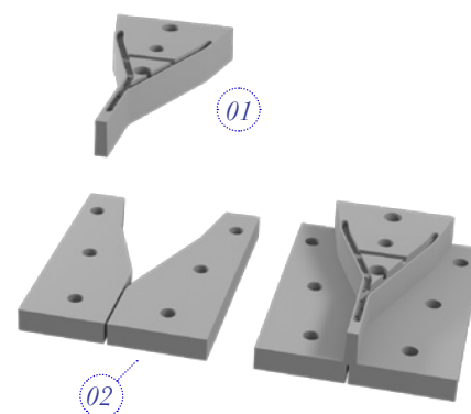
1 / Punch 2 / Die set
